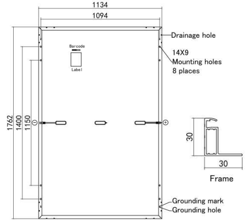
Back side(mm)
